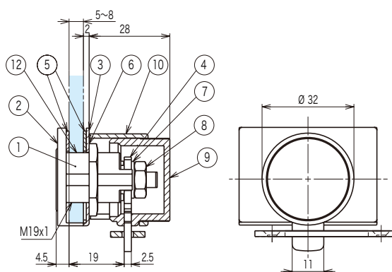
A-A dimension
