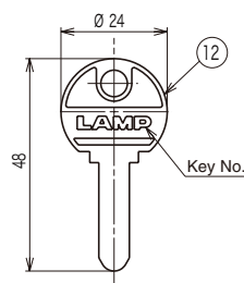
A-A dimension
