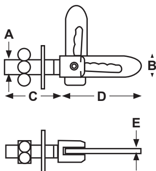
IR67 Anti-Luce Fastening Lug
