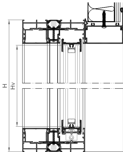
SECCIÓN B-B SECTION B-B
