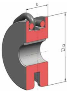
Type A: plain
