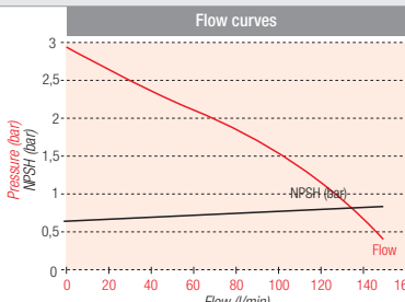
BAG-800 230-400VAC
