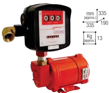
SAG-500
