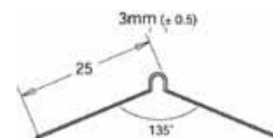
MMG 28mm Mini Mesh Bead
