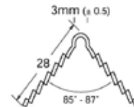
LMG 32mm Mini Mesh Bead
